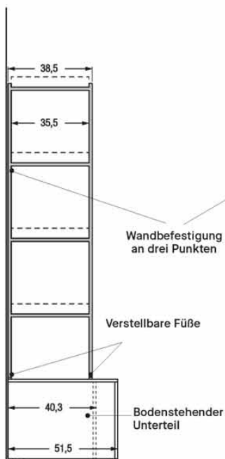
AUFGESETZTER RAHMEN
