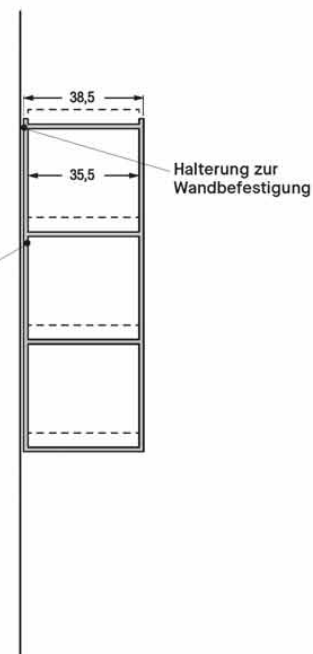
HÄNGERAHMEN
