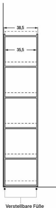
BODENSTEHENDER RAHMEN
